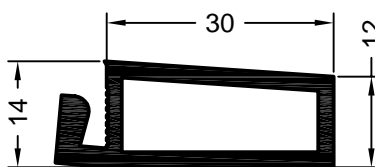
art. 561330 01 jednostka opakowaniowa: 144 m art. 597400 okleinowany jednostka opakowaniowa: 36 m profil poszerzający
