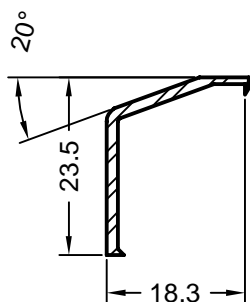
art. 248786 naturalny eloksalowany aluminium jednostka opakowaniowa: 6 m ostona progów 2
