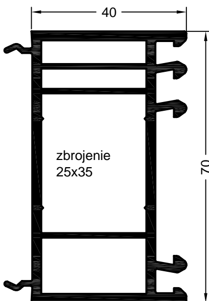
art. 550140 01 art. 599140 okleinowany jednostka opakowaniowa: 36 m poszerzenie ościeżnicy 40/70
