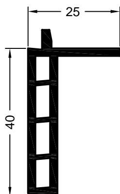
art. 560970 01 jednostka opakowaniowa: 96 m art. 595050 okleinowany jednostka opakowaniowa: 36 m poszerzenie do art. 561670 (prowadnica rolety 1) art. 619589 (prowadnica rolety 2) art. 625533 (prowadnica rolety 3)
