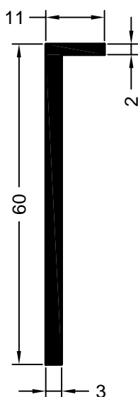
art. 758360 01 jednostka opakowaniowa: 144 m profil licowy 3
