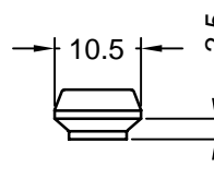
art. 264230 jednostka opakowaniowa: 1000 sztuk kołek do przykręcania
