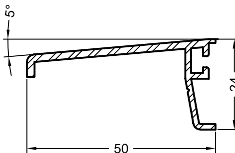
art. 248796 naturalny eloksalowany aluminium jednostka opakowaniowa: 6 m szyna siodłowa z rowkiem pod uszczelkę
