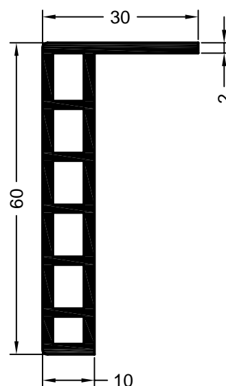
art. 560210 01 art. 593570 okleinowany jednostka opakowaniowa: 72 m profil licowy 4
