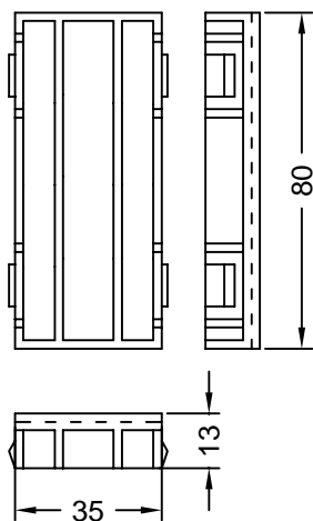
art. 246691 kolor dowolny RAU-PS jedn. opakowaniowa: 100 sztuk podkładka dystansowa 13 do profilu dylatacyjnego 2/70 (skala 1:2)
