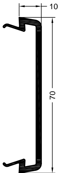
art. 565060 01 art. 585060 okleinowany jednostka opakowaniowa: 36 m poszerzenie ościeżnicy 10/70
