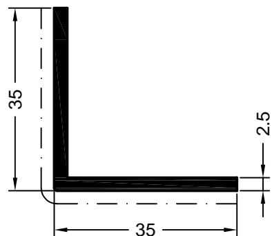
art. 560180 01 jednostka opakowaniowa: 144 m art. 591370 okleinowany jednostka opakowaniowa: 72 m profil narożny 2
