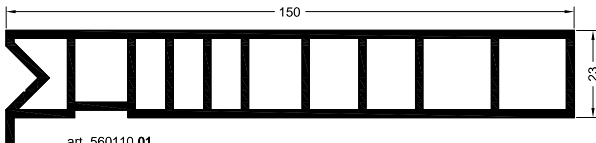
art. 560110 01 jednostka opakowaniowa: 24 m profil prowadzący F do okiennicy składanej
