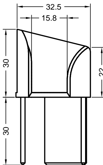
art. 230536 prawy, biały, brązowy art. 230546 lewy, biały, brązowy RAU-ASA jednostka opakowaniowa: 100 sztuk regulator wlotu rolety 3 do przewodnicy rolety 3
