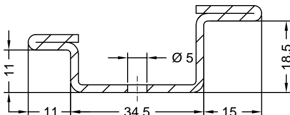
art. 260504 stal ocynkowana zbrojenie do poprzeczniczy rolety 1 jednostka opakowaniowa: 6 m I_x = 13,9 \text{ cm}^4
