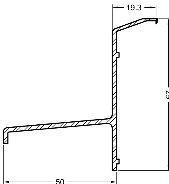
art. 231120 naturalny eloksalowany aluminium jednostka opakowaniowa szyna siodłowa 2/70
