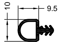
art. 865520 czarny RAU-SR jedn. opakowaniowa: 200 m uszczelka do profilu dylatacyjnego 2/70
