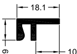
art. 626071 01 jednostka opakowaniowa: 144 m profil do osłony tynku
