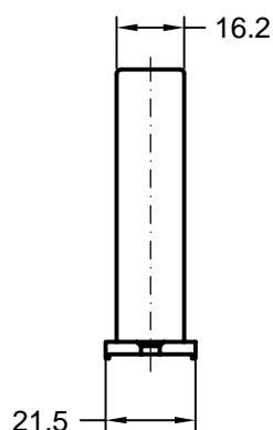
art. 268362 kolor dowolny RAU-PA jednostka opakowaniowa: 100 sztuk łącznik szczeliny do mostka łączącego szczeliny - połączenie krzyżowe
