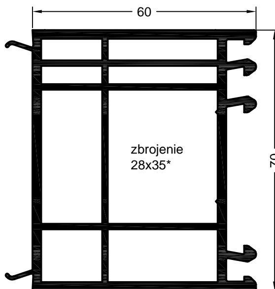
art. 561113 01 art. 597113 okleinowany jednostka opakowaniowa: 36 m poszerzenie ościeżnicy 60/70
