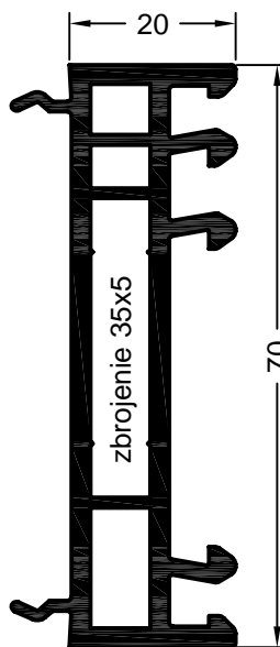
art. 550210 01 art. 599310 okleinowany jednostka opakowaniowa: 36 m poszerzenie ościeżnicy 20/70
