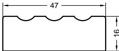
art. 257833 biały RAU-ASA jednostka opakowaniowa: 1 sztuka pokrywka zakończeniowa do profilu dekoracyjnego 1
