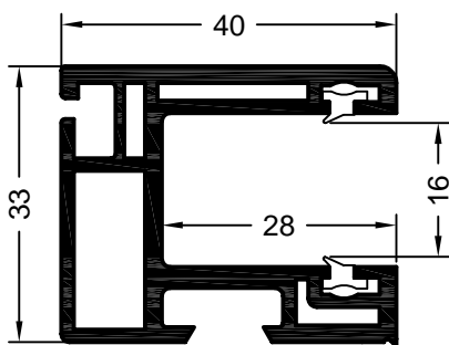
art. 625533 01 jednostka opakowaniowa: 72 m art. 625543 okleinowany jednostka opakowaniowa: 24 m RAU-PVC/PREN przewodnica rolety 3
