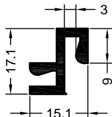
art. 625171 01 jednostka opakowaniowa: 144 m profil łączący
