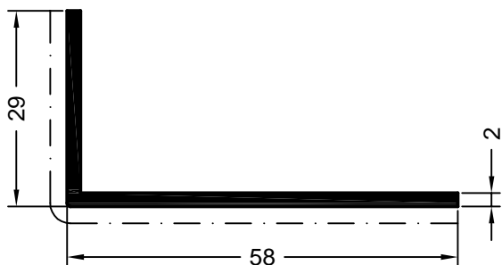
art. 560190 01 jednostka opakowaniowa: 144 m art. 591340 okleinowany jednostka opakowaniowa: 72 m profil narożny 1
