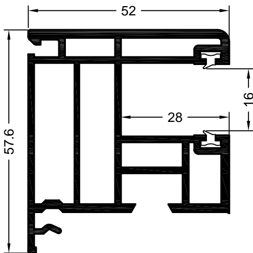
art. 619589 01 RAU-PVC/PREN jednostka opakowaniowa: 36 m przewodnica rolety 2
