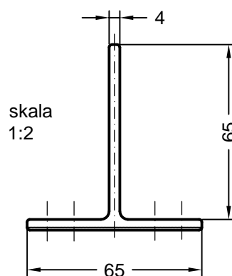
art. 268362 kolor dowolny RAU-PA jednostka opakowaniowa: 100 sztuk łącznik szczeliny do mostka łączącego szczeliny - połączenie krzyżowe
