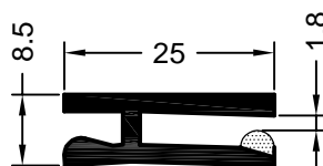
art. 733020 05 jednostka opakowaniowa: 144 m art. 590160 okleinowany jednostka opakowaniowa: 72 m RAU-PVC/PREN profil podtrzymujący płyty
