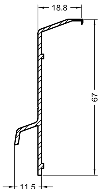
art. 222700 naturalny eloksalowany aluminium jednostka opakowaniowa: 6 m szyna siodłowa 1/70
