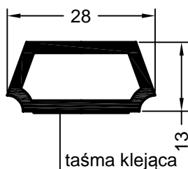
art. 560530 01 jednostka opakowaniowa: 144 m art. 593700 okleinowany jednostka opakowaniowa: 72 m szczelina 1
