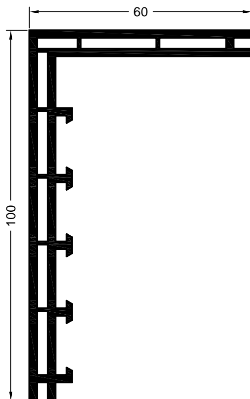
art. 606252 01 art. 591280 okleinowany jedn. opakowaniowa: 36 m profil licowy 1
