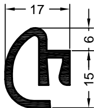
art. 561700 01, brązowy jednostka opakowaniowa: 144 m poprzecznicza rolety 1
