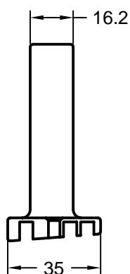
art. 268352 kolor dowolny RAU-PA jednostka opakowaniowa: 100 sztuk łącznik szczeliny do mostka łączącego szczeliny - wrąb szyby
