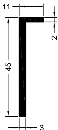
art. 758370 01 jednostka opakowaniowa: 144 m profil licowy 2
