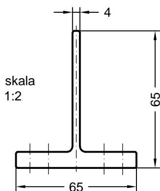
art. 268352 kolor dowolny RAU-PA jednostka opakowaniowa: 100 sztuk łącznik szczeliny do mostka łączącego szczeliny - wrąb szyby
