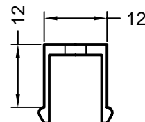
art. 258690 aluminium jedn. opakowaniowa: 100 sztuk zacisk
