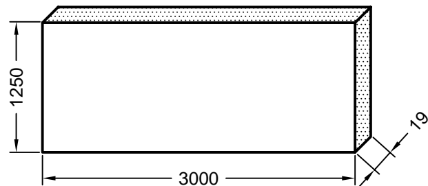
art. 901223 3000x1250x19 mm U = 2,1 W/m 2 K jednostka opakowaniowa: 1 sztuka
