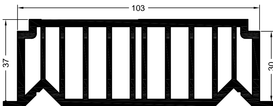
art. 560110 01 jednostka opakowaniowa: 24 m profil prowadzący F do okiennicy składanej
