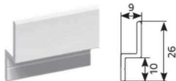
Profilé de la glissière type « Z »
