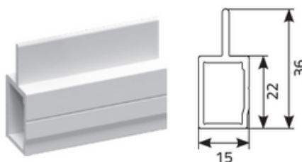
profilé de la glissière type « F1 »
