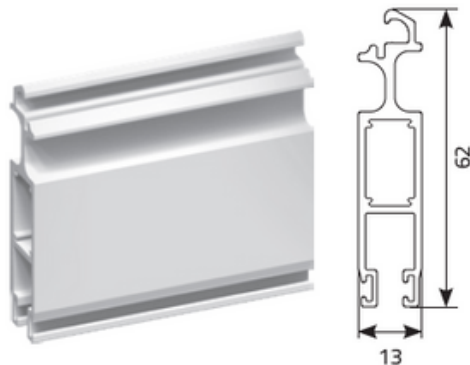
Profilé du cadre « MPR »
