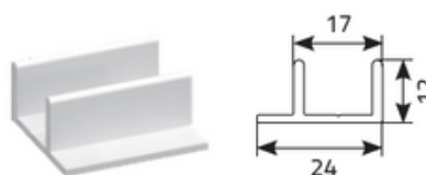
Profilé de la glissière type « U »
